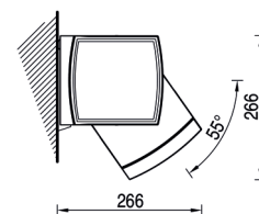
Installazione a parete 55°
