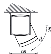
Installazione a soffitto 65°
